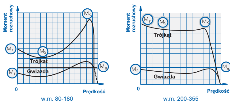
Wykres zależności momentu rozruchowego od prędkości
