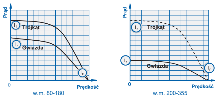
Wykres zależności prądu od prędkości
